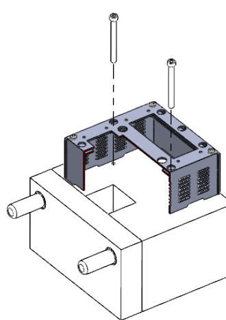
Fixação molde - opção 2 Mold fixation - option 2
