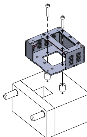
Fixação molde - opção 2 Mold fixation - option 2
