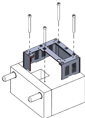
Fixação molde - opção 1 Mold fixation - option 1
