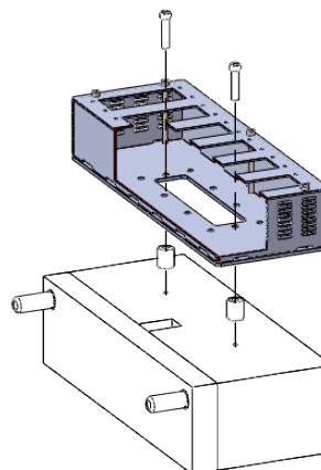
Fixação molde - opção 2 Mold fixation - option 2
