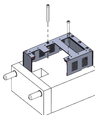
Fixação molde - opção 2 Mold fixation - option 2
