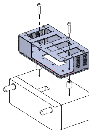
Fixação molde - opção 2 Mold fixation - option 2
