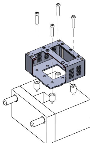
Fixação molde - opção 1 Mold fixation - option 1
