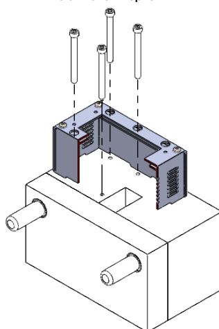
Fixação molde - opção 2 Mold fixation - option 2
