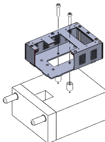
Fixação molde - opção 2 Mold fixation - option 2
