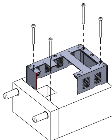
Fixação molde - opção 1 Mold fixation - option 1
