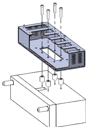
Fixação molde - opção 1 Mold fixation - option 1
