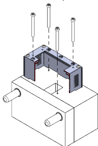
Fixação molde - opção 1 Mold fixation - option 1
