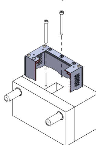
Fixação molde - opção 3 Mold fixation - option 3
